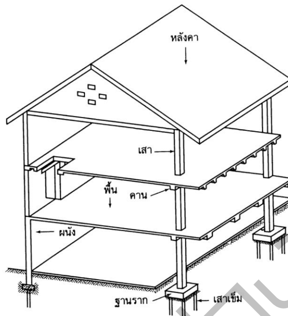
ภาพที่ 1.1 ส่วนประกอบโครงสร้างต่างๆของอาคาร ที่มา (สิทธิโชค สุนทรโอภาส, 2543, หน้า 16)
